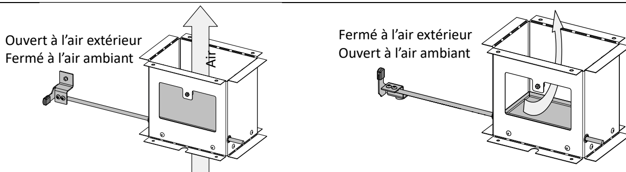
Figure 24 Fonctionnement du contrôle d'air extérieur
