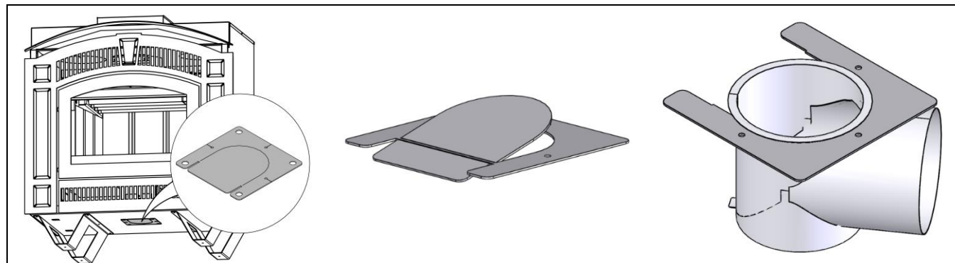
Figure 7 Couvercle d'air extérieur
