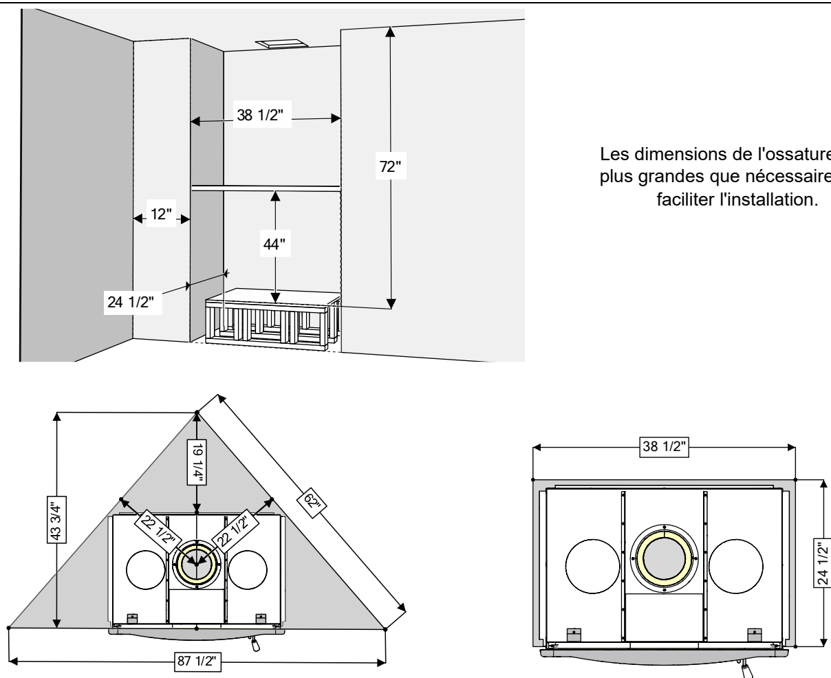
Figure 4 Exemples d'ossature pour le PERLE 3600B
