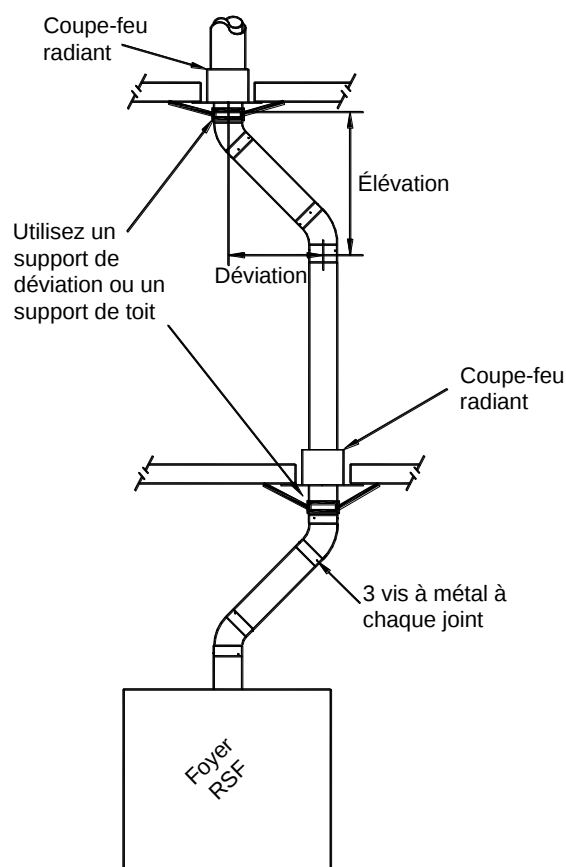
Figure 14 Exemple d'installation d'une cheminée avec déviation
