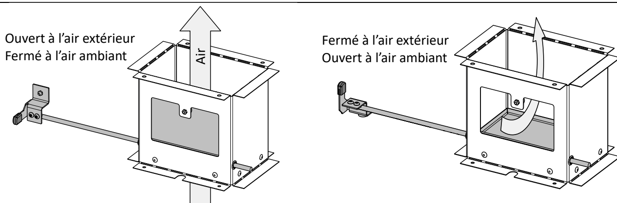
Figure 25 Fonctionnement du contrôle d'air extérieur
