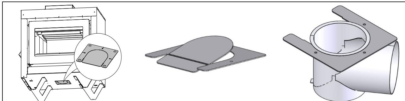
Figure 7 Couvercle d'air extérieur
