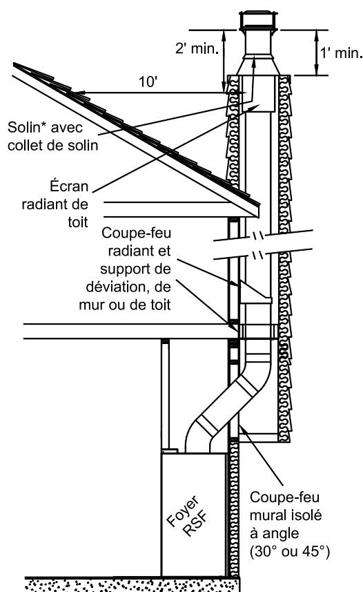
Figure 15 Exemple d'installation à travers le mur
