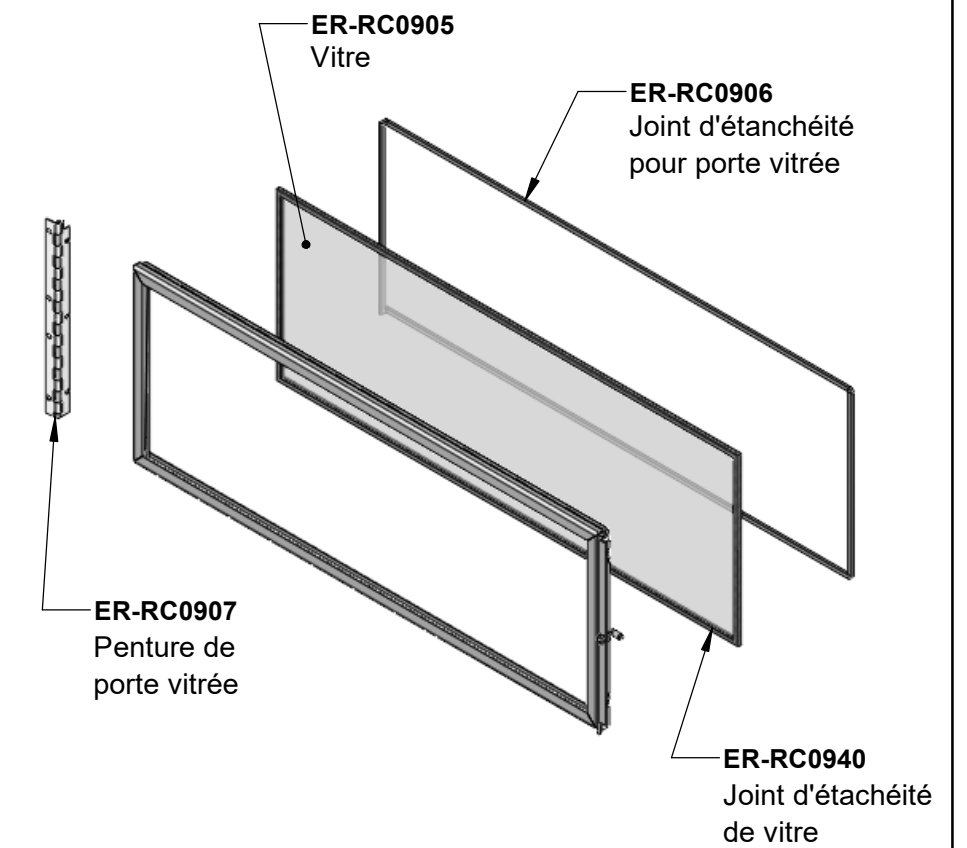
ER-RC0908 Porte vitrée assemblée
