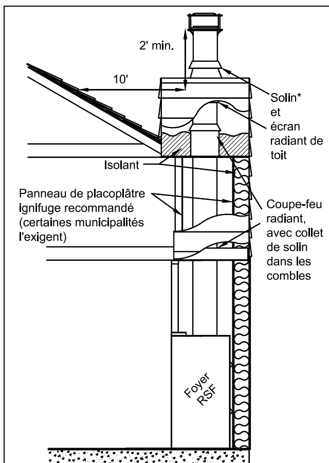
Figure 10 Exemple d'installation d'une cheminée encloisonnée
