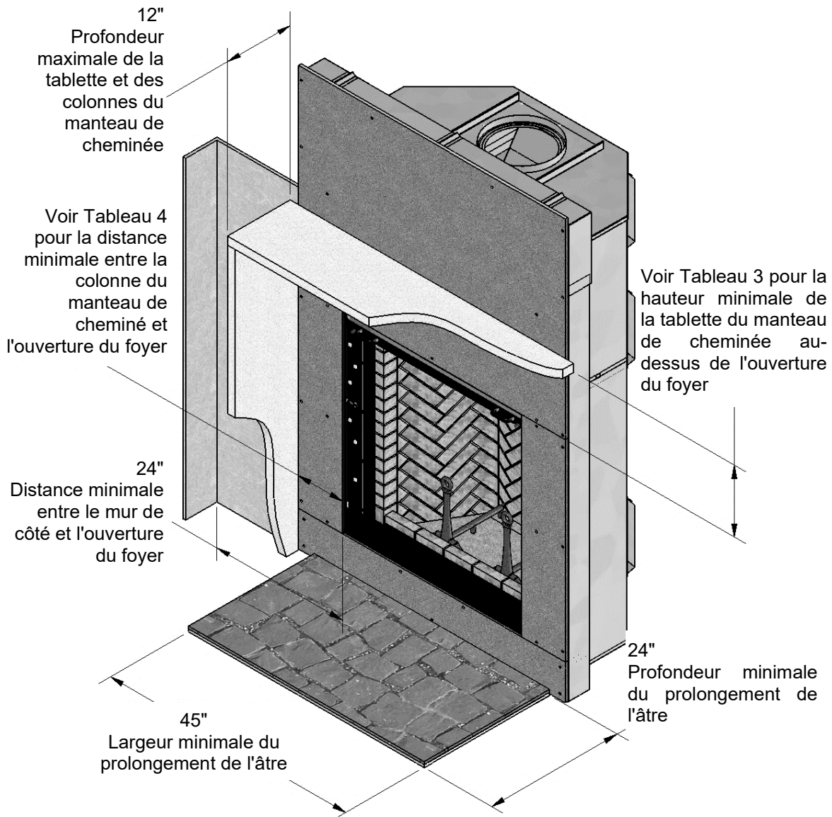
FIGURE 8 DÉGAGEMENTS DU FOYER (VOIR TABLEAU 2)
