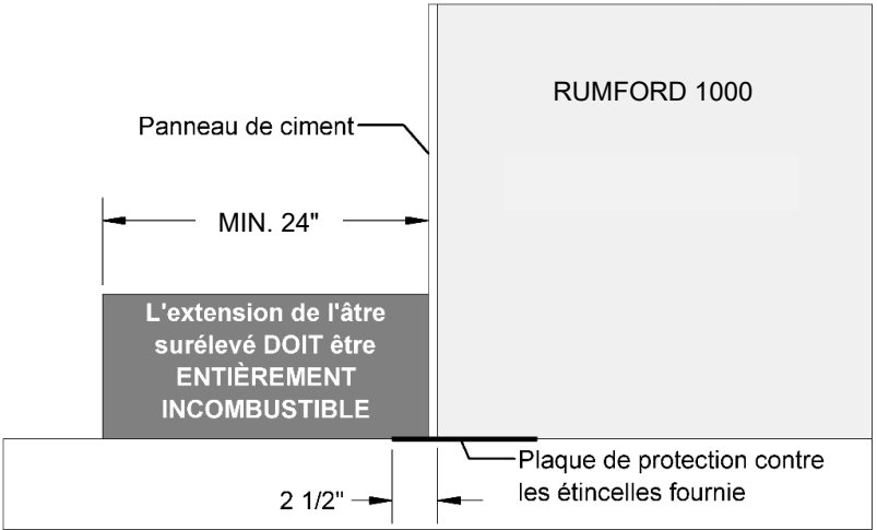
FIGURE 11 DIMENSIONS MINIMUM DE L'EXTENSION DE L'ÂTRE
