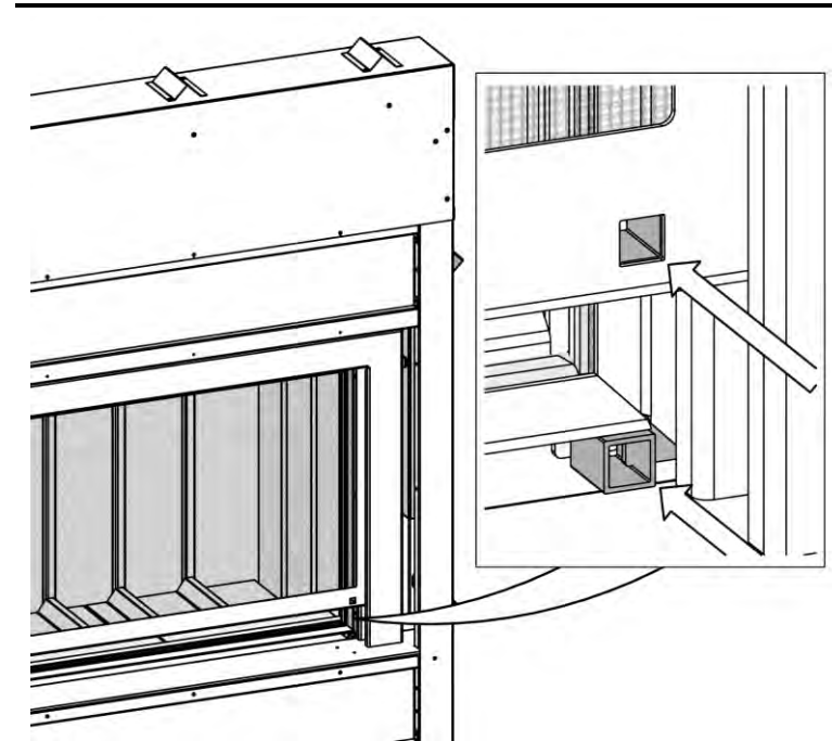
Figure 1 Emplacement de l'œillet de la poignée de porte et du pare-étincelle
