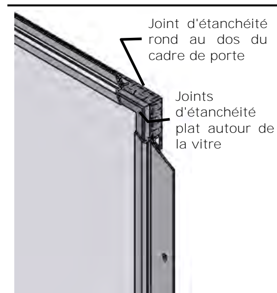
Figure 3 Côté droit de la porte vitrée
