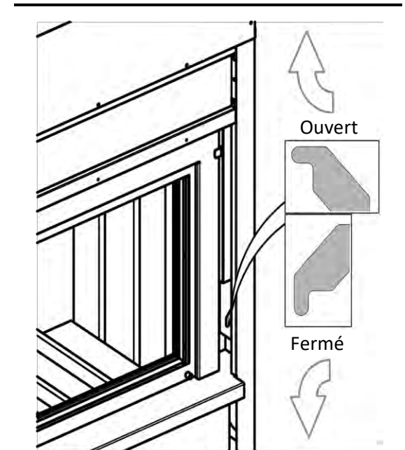
Figure 2 Contrôle d'air extérieur
