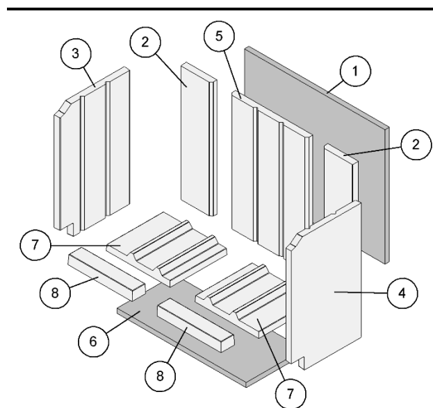
Figure 4 Pierres réfractaires et panneaux d'isolant
